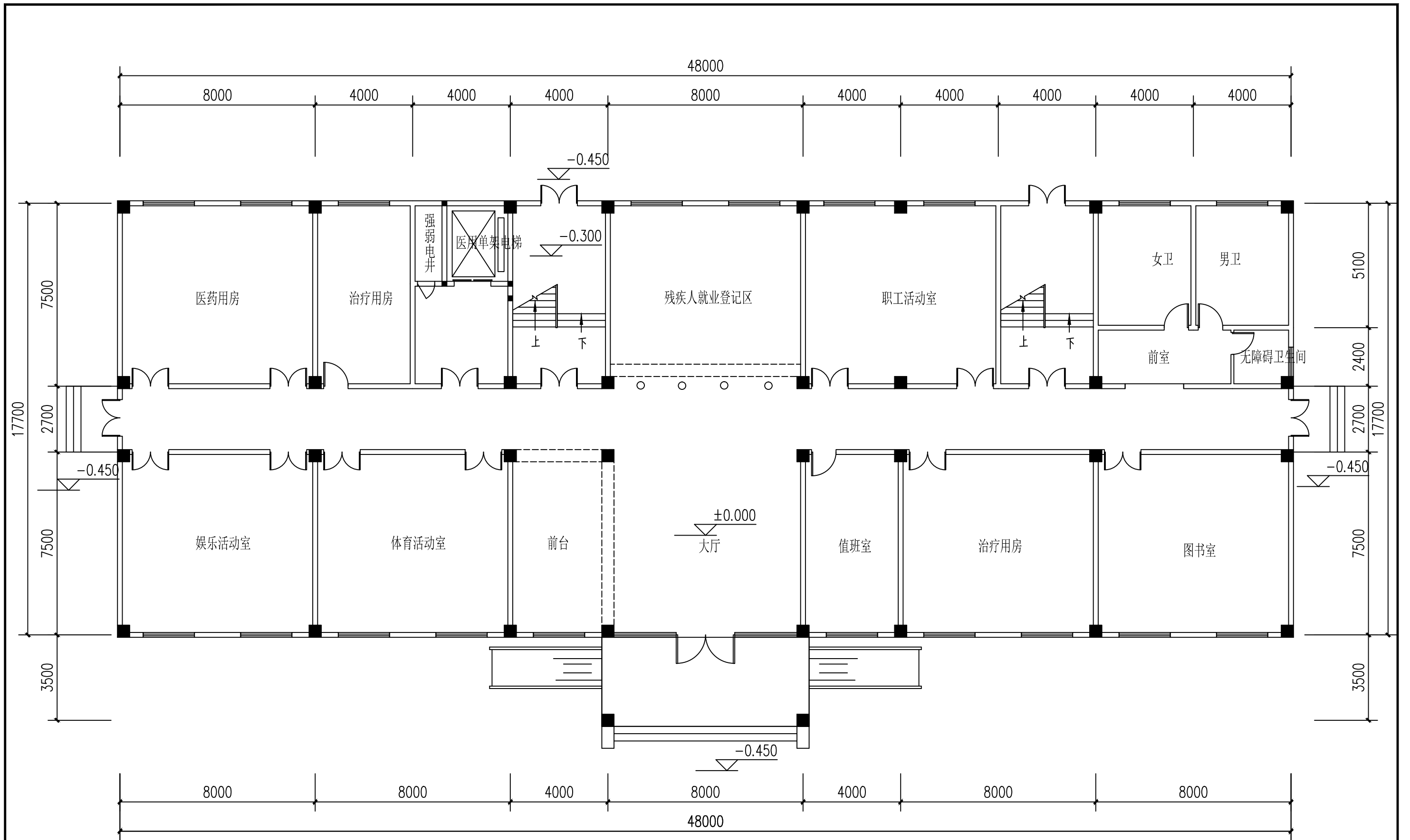
一层平面图 1:150
