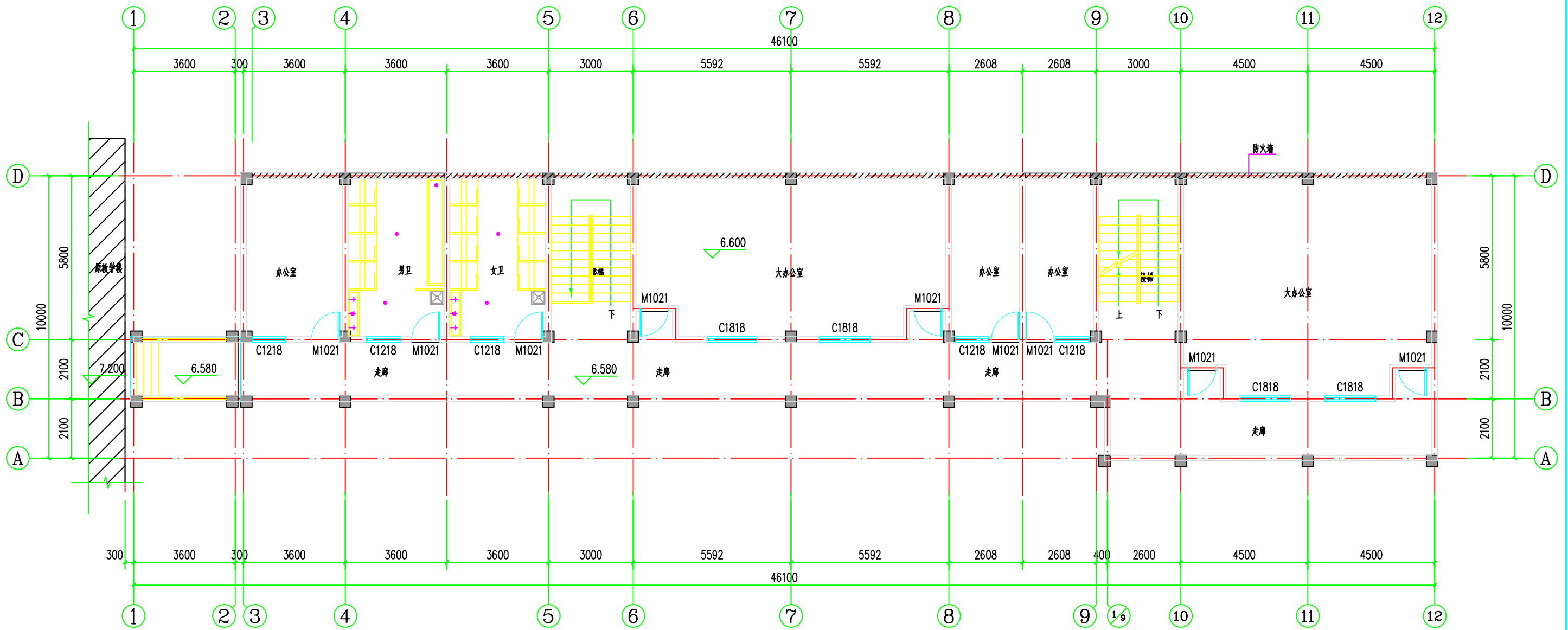
三层平面图 1:100
