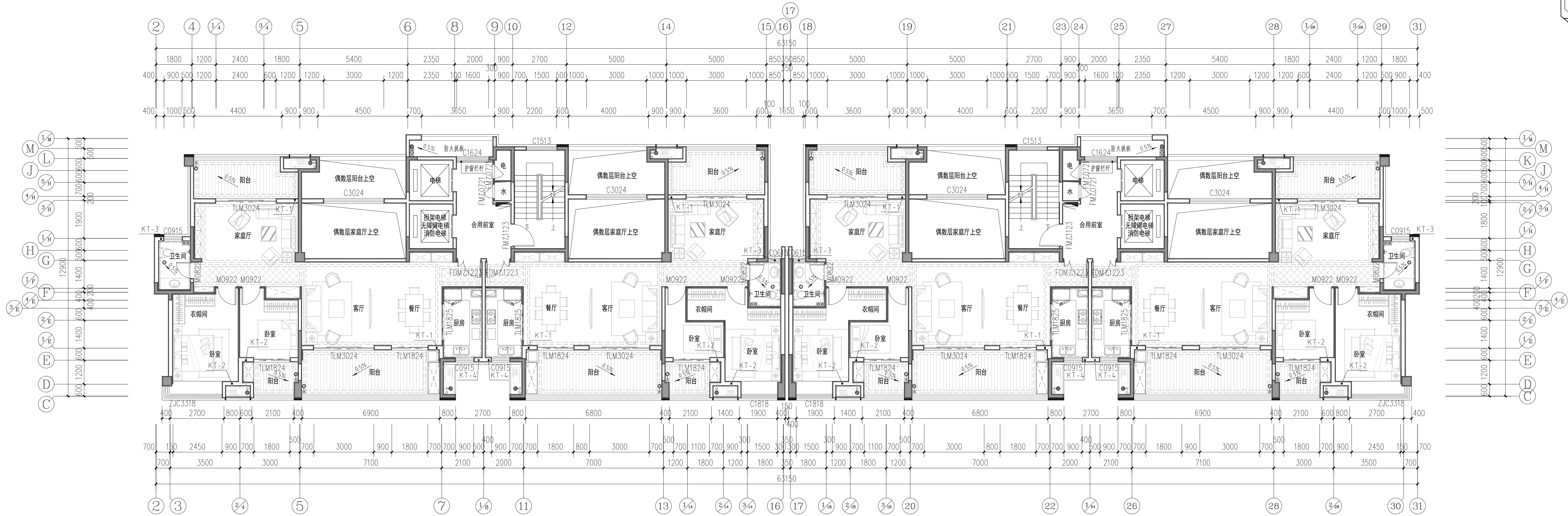
3#、4#楼标准层平面图(奇数层) 1:100
