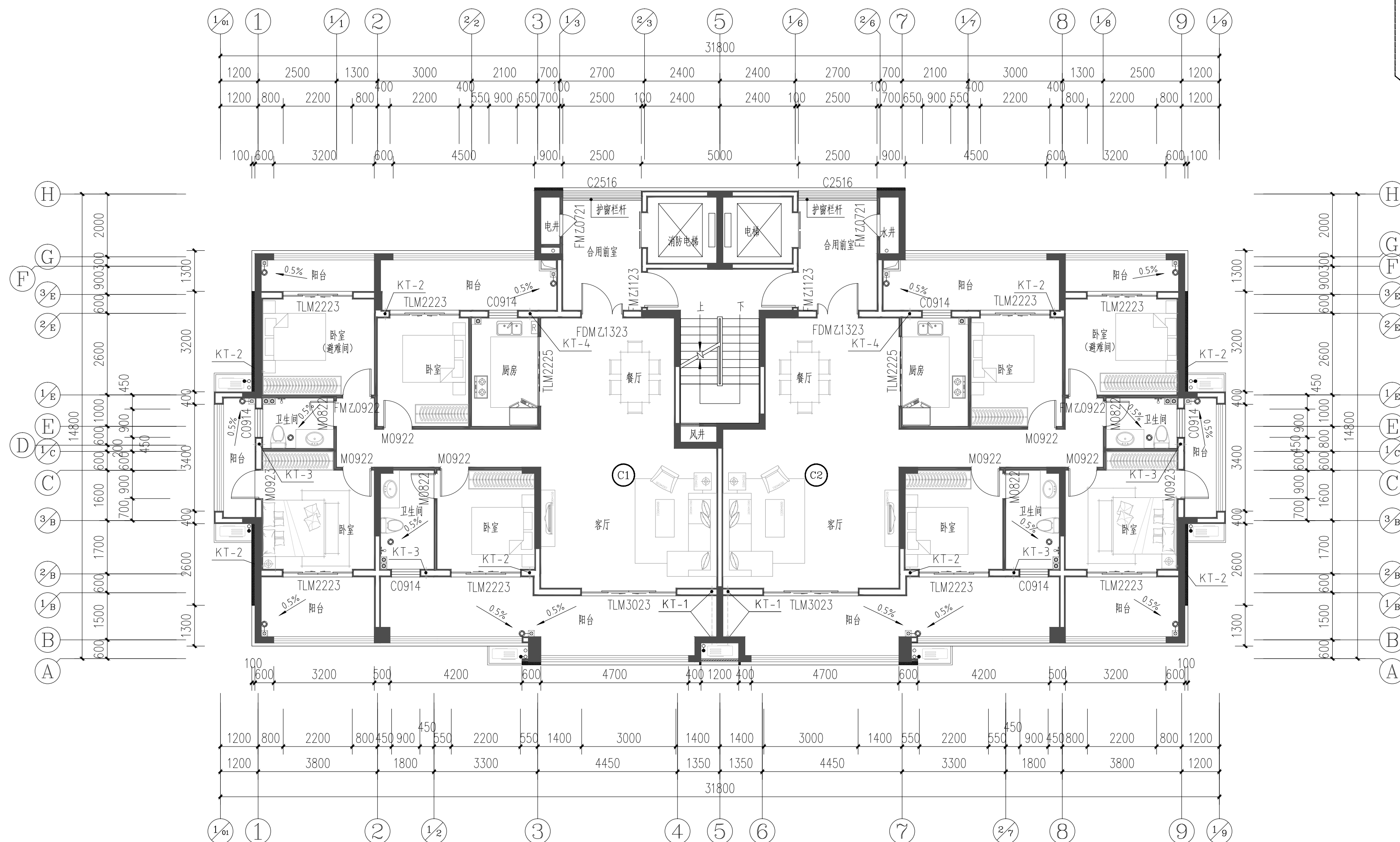
5#楼标准层平面图 1:100
