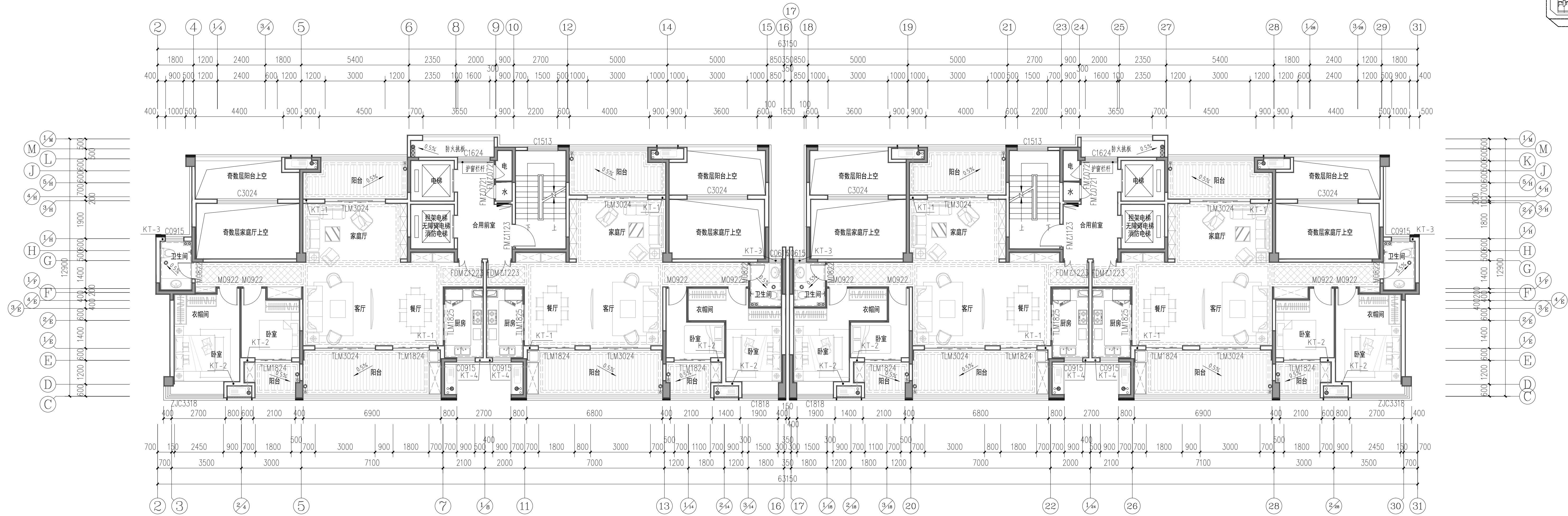
3#、4#楼标准层平面图(偶数层) 1:100
