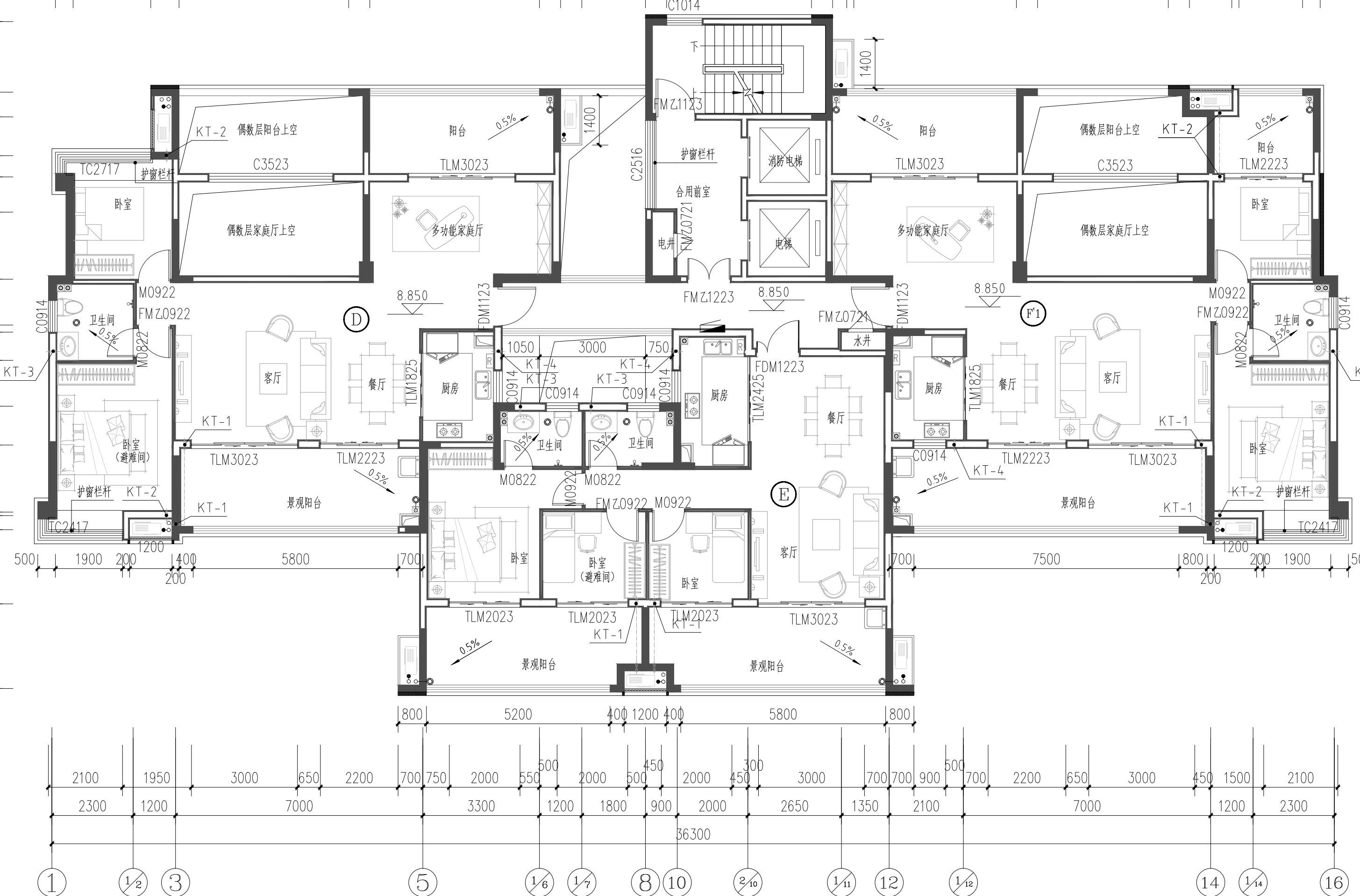
8#、9#、10#楼标准层平面图(奇数层) 1:100
