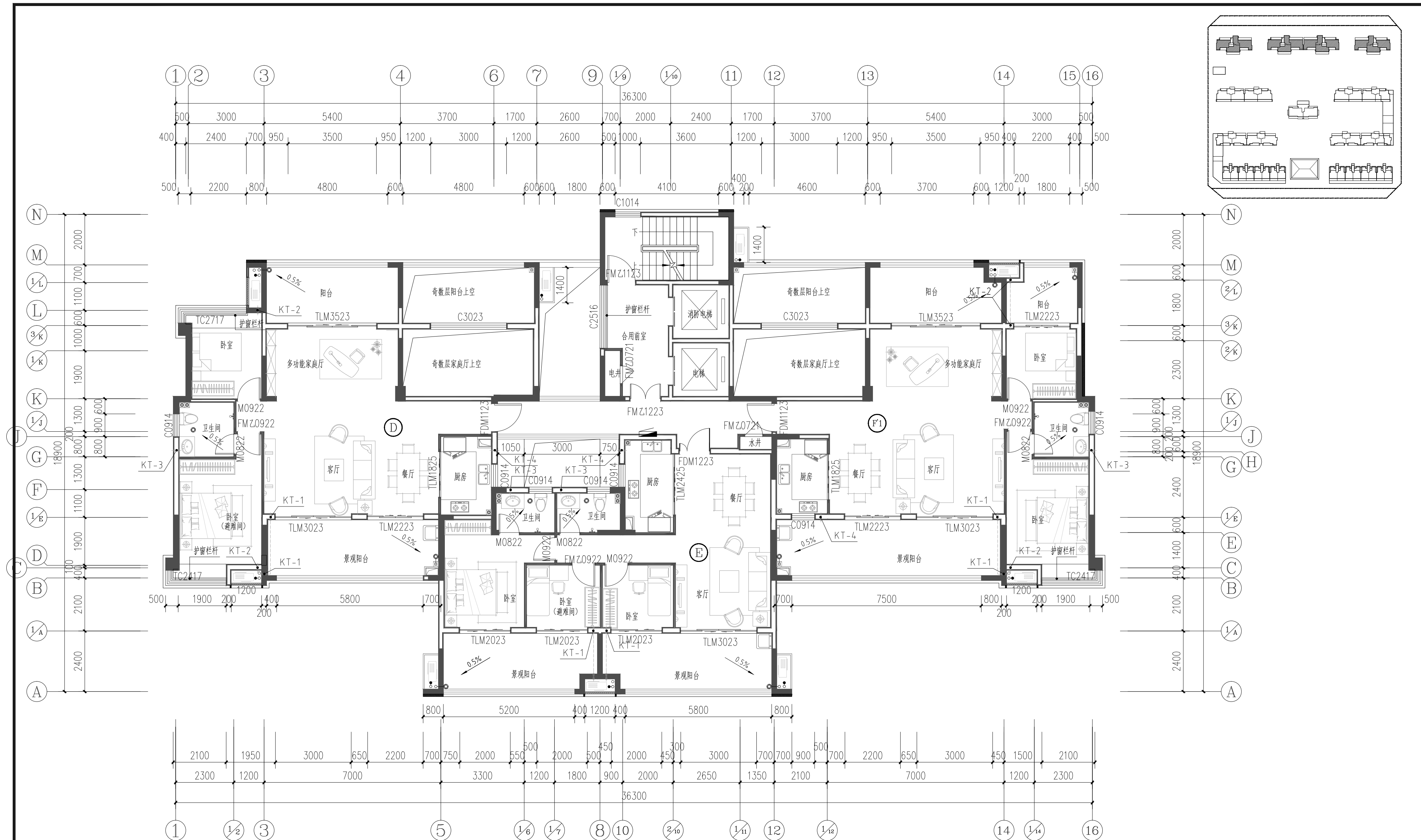
8#、9#、10#楼标准层平面图(偶数层) 1:100
