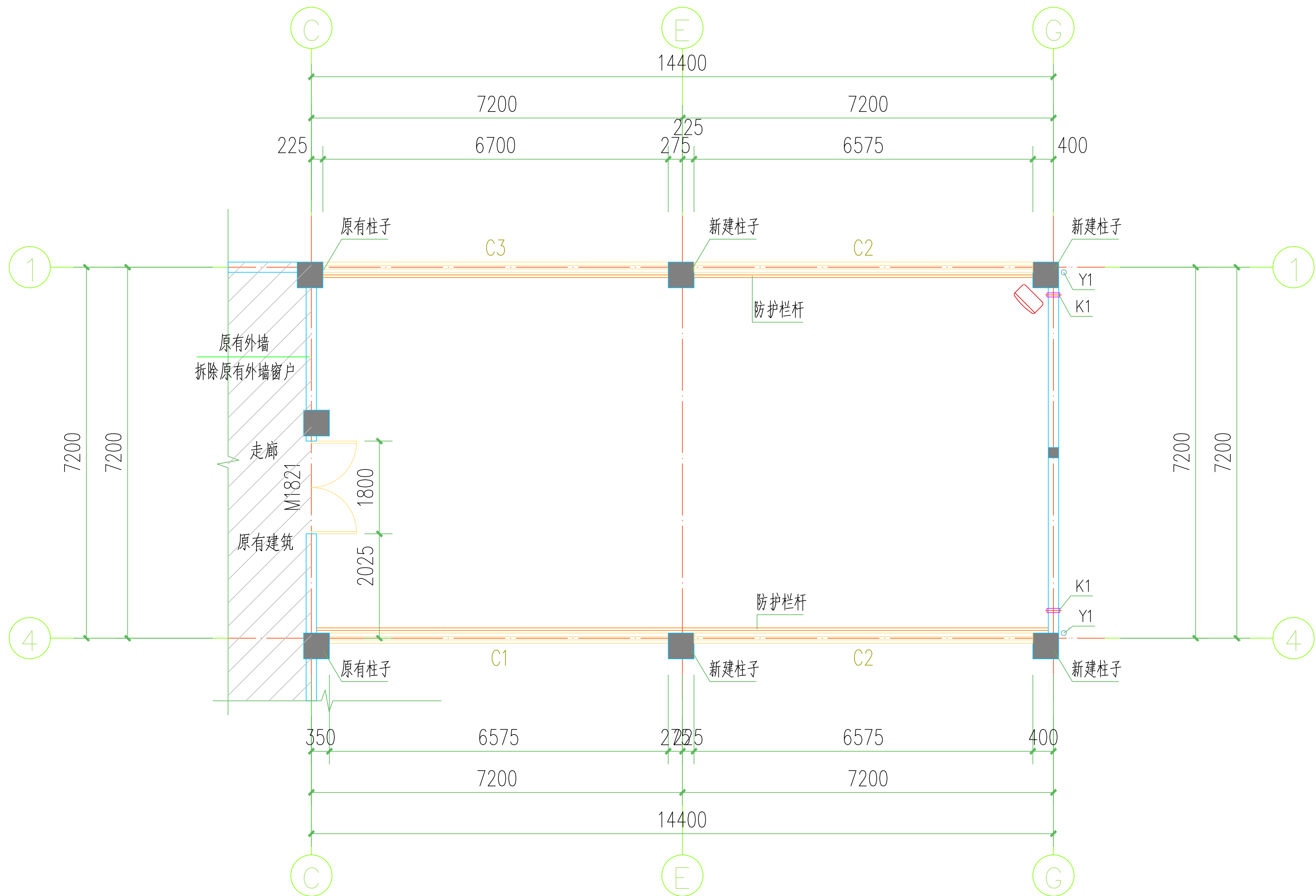
五层局部平面图 1:100
